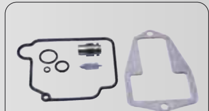
Varenr.: 226202 Ref. nr. CAB-S3 Ventil-sæt 133370-44500 (13370-27A00) Pakning FBG-301 Pakning 13266-27A00 Oringe
